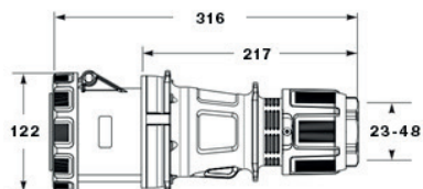
Tomada reta de embutir reta IP67
