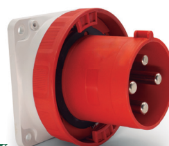
Plugue de embutir IP67
