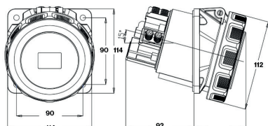
Tomada de bloqueio mecânico IP67
